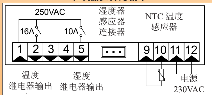
湿度器控制线路图
